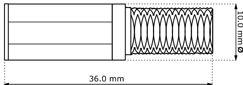
Steckergehäuse mit Knickschutz cover with cable protection
