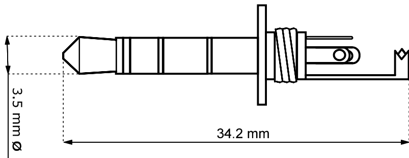
Stecker plug
