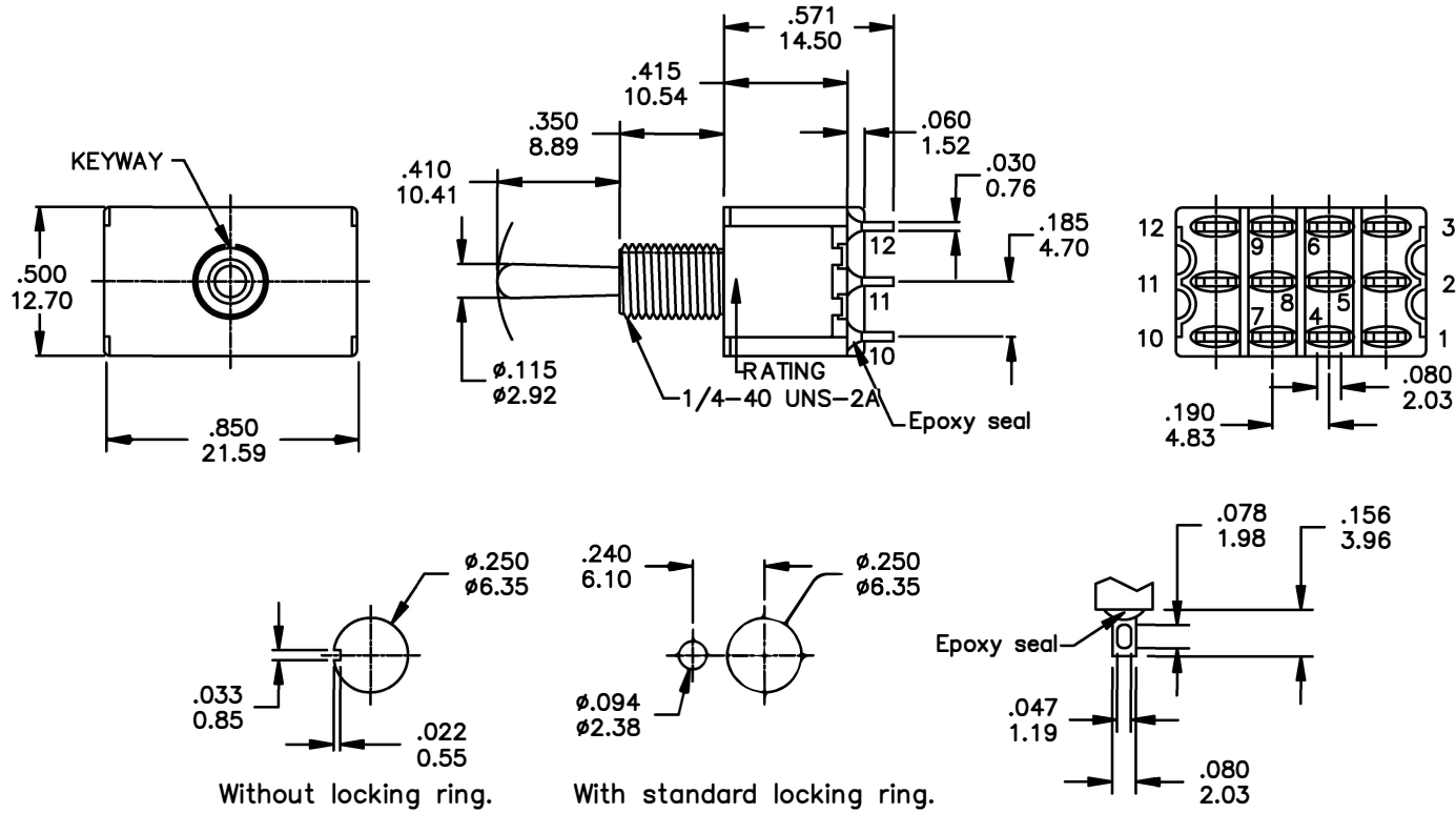
SOLDER LUG
