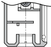
Maze strain relief Labyrintdragavlastning
